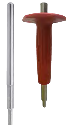
内迫膨胀锚栓安装工具
